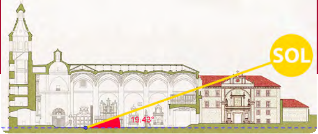
El rayo solar que cruza la ventana occidental y el gnomon del trancoro, se proyecta en el centro de la iglesia
